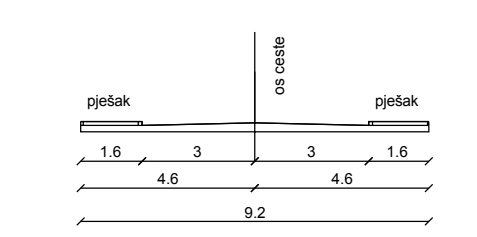
KARAKTERISTIČAN POPREČNI PRESJEK B-B MJ. 1:200
