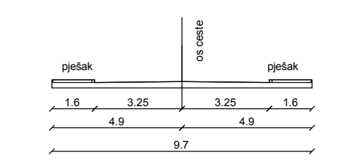
KARAKTERISTIČAN POPREČNI PRESJEK B-B MJ. 1:200
